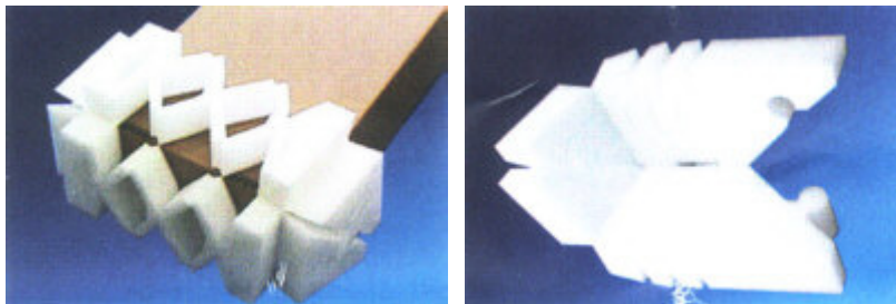
Flexible Doppel-Clip Ecke aus TechnoFoam®-Plus. Es werden nur 4 Ecken für eine Verpackung gebraucht.
